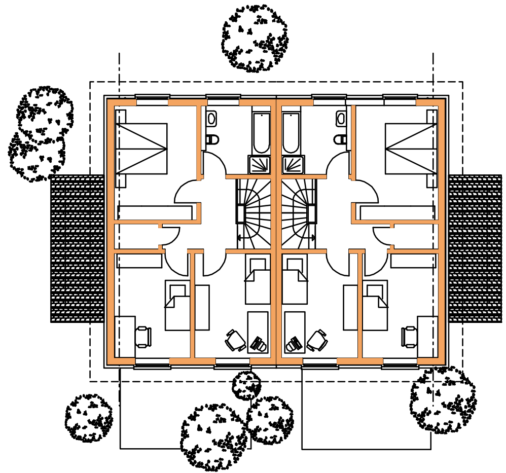
GRUNDRISS DACHGESCHOSS
