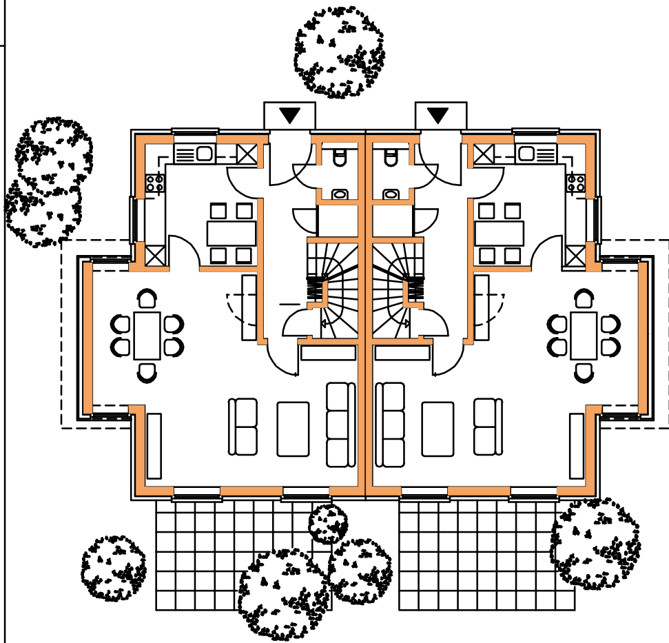
GRUNDRISS ERDGESCHOSS
